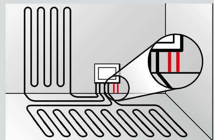
Nachher: platzsparende Flächentemperierung an Wand und Boden mit der Kleinflächenregelstation. Optimal für die Renovierung einzelner Räume. Die Kleinflächenregelstation wird einfach an bestehende Heizkörperanschlüsse angeschlossen.
